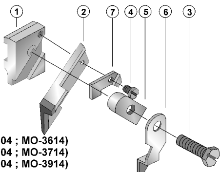
118-23804 Perno
