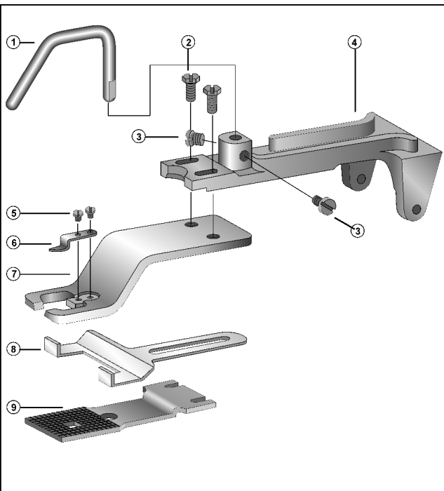
MAT-61401ZB0 Pinza per etichette cpl.
