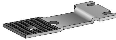
B2529-372-B00 Placca liscia per bottone piccolo (MB-372)
