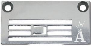
Placca 2 aghi Needle plate (2 needles) cod. E1524 (2x4,0 mm) cod. E1525 (2x4,8 mm)
