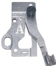
Gruppo coltelli cpl. Knives group asm. cod. 925891-4-00
