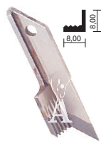
Coltello sup. widia dentato Upper knife widia for knitting cod. 207002-2-00 (v.t.) cod. 209357-2-01 (n.t.)
