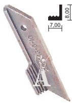
Coltello sup. dentato Upper knife for knitting cod. 202143-0-10 (v.t.) cod. 209350-0-00 (n.t.)
