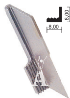
Coltello sup. dentato Upper knife for knitting cod. 203010-0-10 (v.t.) cod. 209358-0-00 (n.t.)
