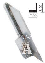
Coltello sup. widia dentato Upper knife widia for knitting cod. 207008-2-00 (v.t.) cod. 209349-0-00 (n.t.)
