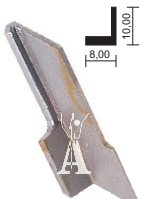
Coltello sup. Upper knife cod. 203783-0-10 (v.t.) cod. 209352-0-00 (n.t.)
