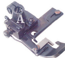
Piedino 2 aghi Presser foot (2 needles) cod. 304408-0-10 (2,0/2,5 mm) cod. 304407-0-10 (3,0/3,5 mm) (= 306679-3-00)
