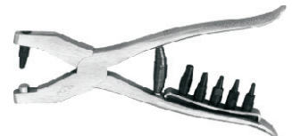
Fustellatrice Hollow puncher
