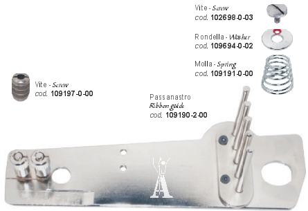
Piastra vibrante - Binder set plate
