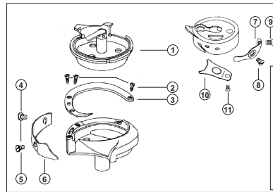
cod. 0167 150270 (alluminio - aluminium)
