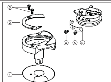
cod. 0249 000378 (metallo - metal)
