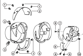
cod. 0069 005800 (metallo - metal)
