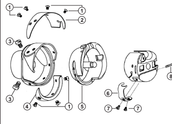
cod. 0069 005800 (metallo - metal)
