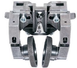
Gruppo piedino a rotelle molleggiato Bouncing roller feet group cod. 102/RTM
