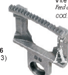
Griffa due aghi - Feed dog (2 needles) cod. 0268 212090 (1,2 - 1,6 mm) (= 0268 212020) cod. 0268 212100 (2,0 - 2,4 mm) (= 0268 212030)
